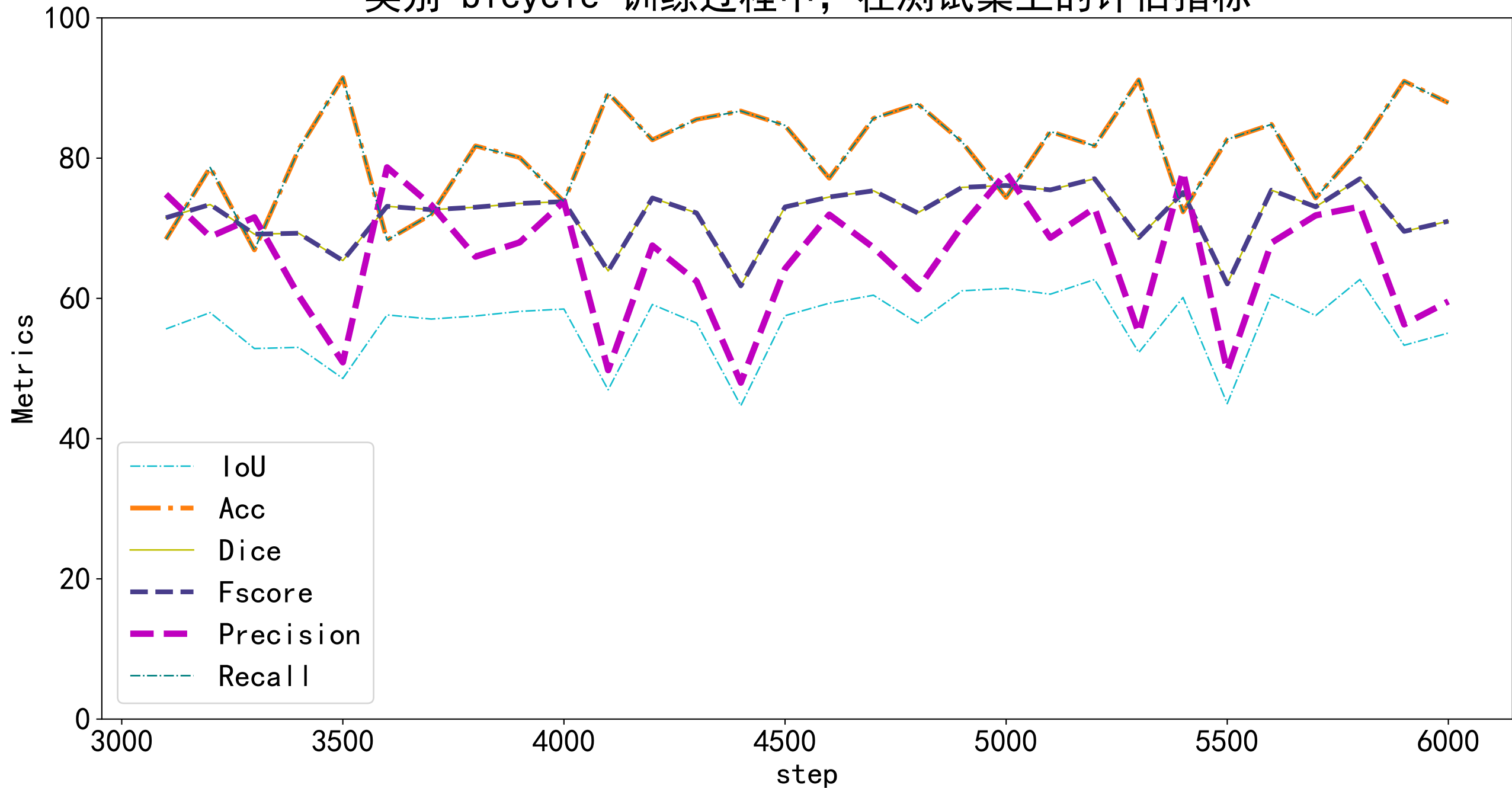
类别 bicycle 训练过程中，在测试集上的评估指标
